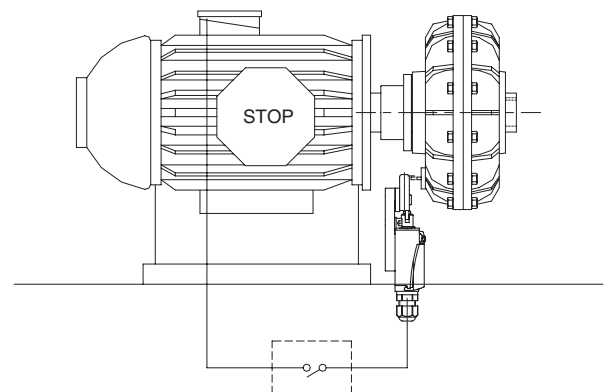
DISPOSITIVO "ET" IMPIEGATO PER ARRESTO MOTORE
