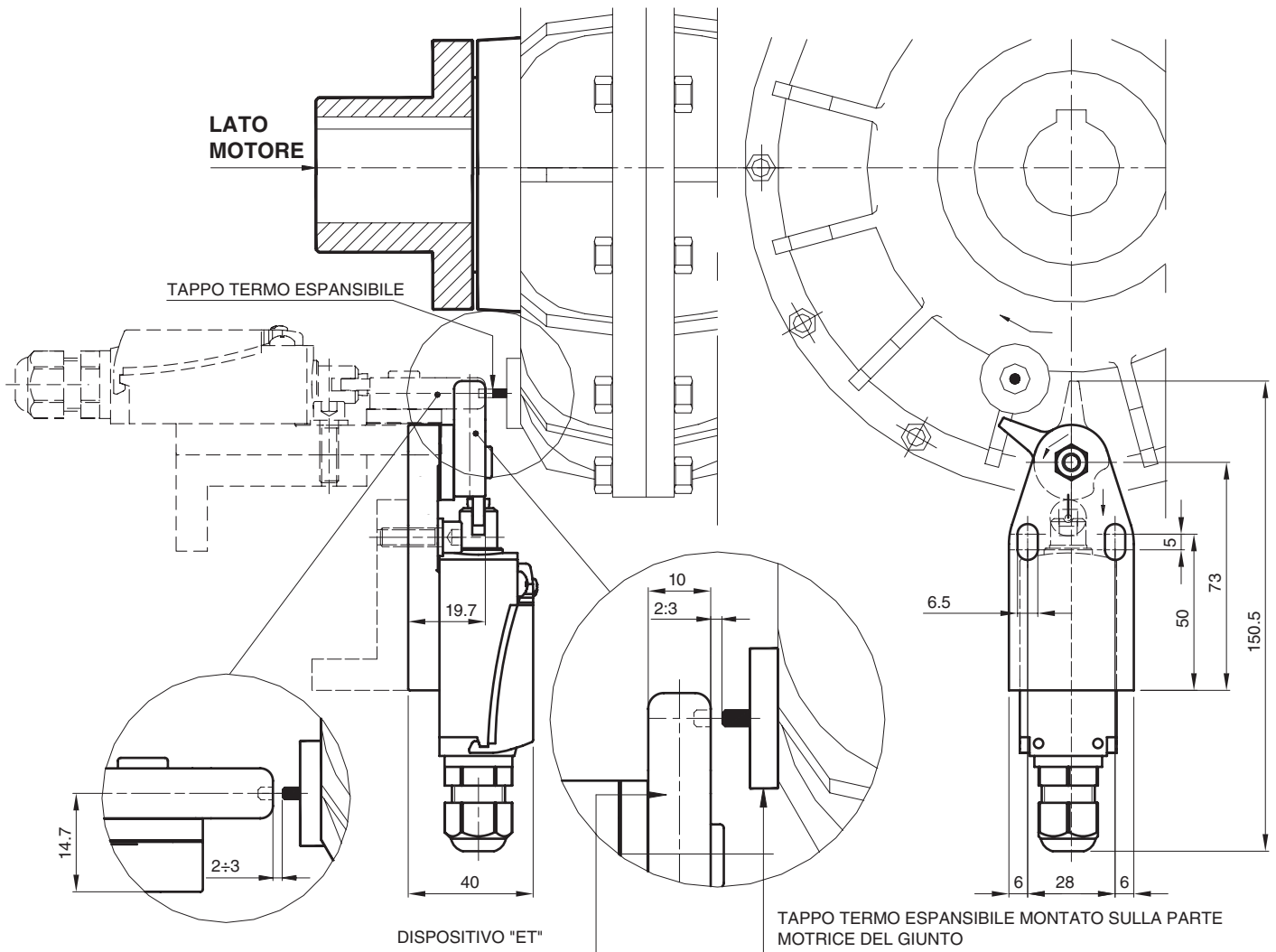
DISPOSITIVO "ET" COLLEGATO AD ALLARME
